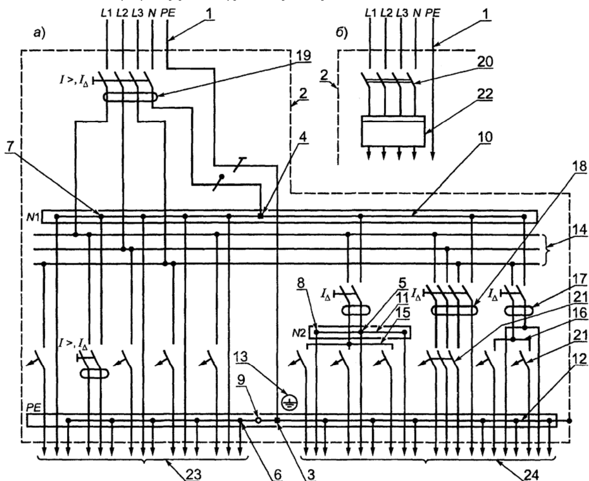
Рисунок А.4 — Схема квартирного группового щитка (для хозблока), присоединенного к квартирному учетно-групповому щитку жилого дома
